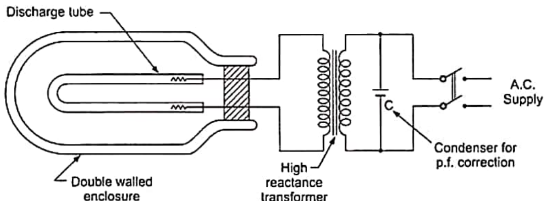
Fig. 7 Sodium vapour lamp
